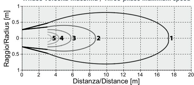
Trifase velocità massima / Three-phase maximum speed
